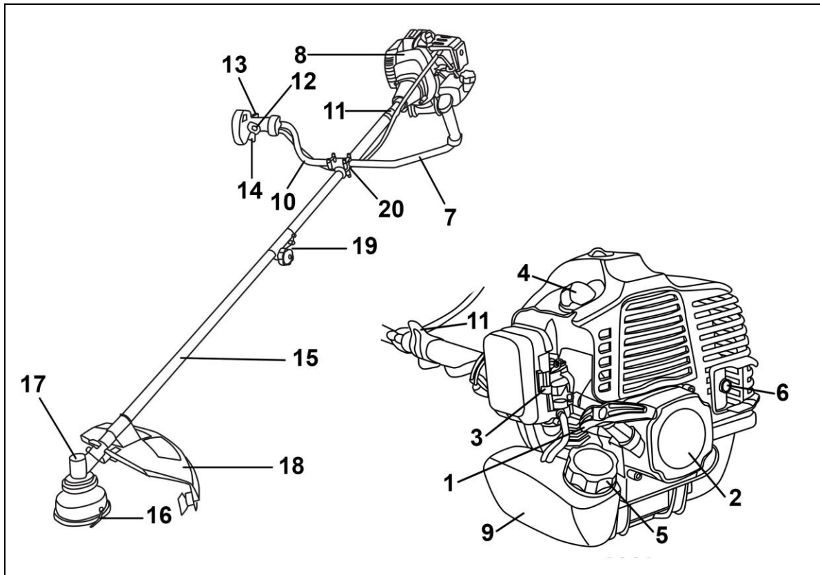
Рис. 1. Общий вид
